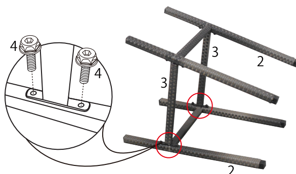
④六角穴付フランジボルト M6×15
